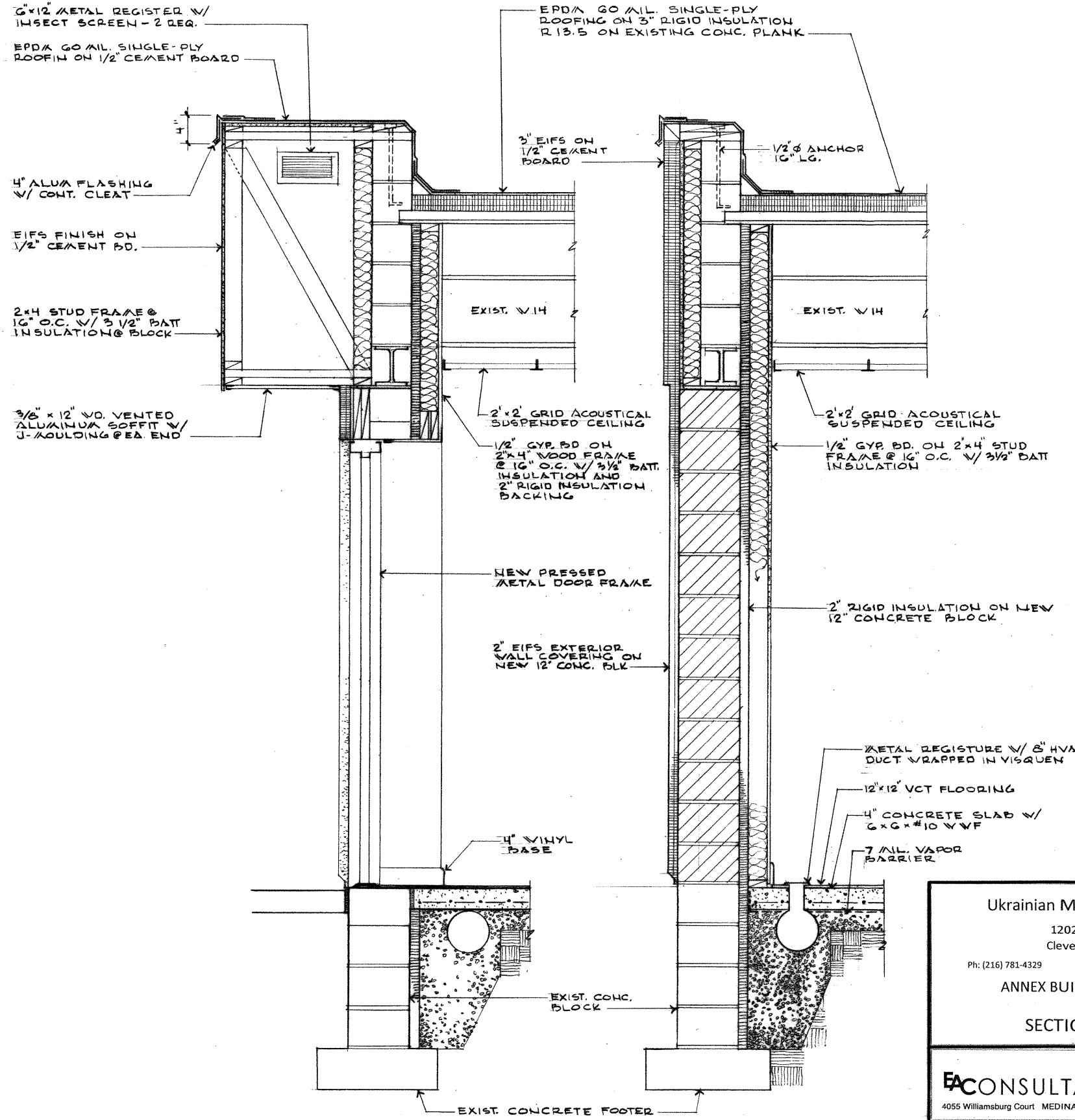
WALL SECTION 'D' SCALE: 1" = 1'-0" WALL SECTION 'C' SCALE: 1" = 1'-0"
